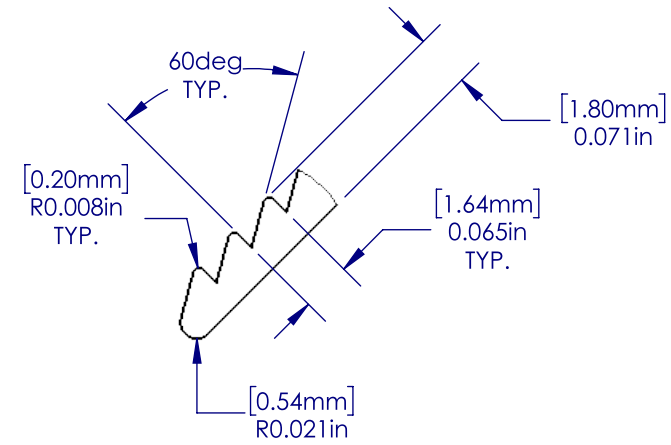
SCALE 4:1
